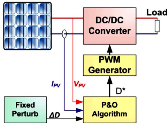
شکل ۱۸: طرح کلی روش تعدیل یافته P&O
