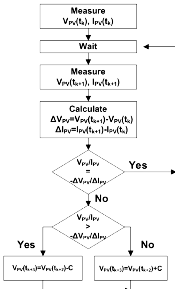
شکل ۲۴: فوچارت روش IC
