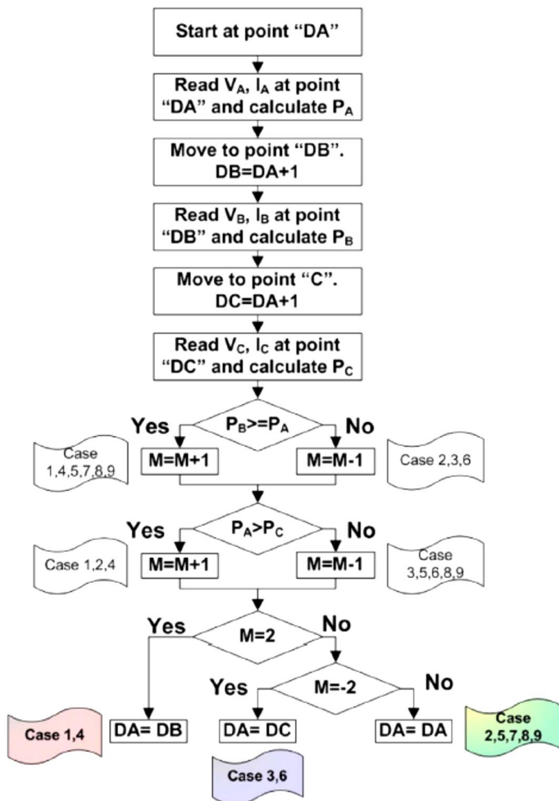
شکل ۲۱: فلوچارت روش مقایسه‌ی وزنی ۳ نقطه‌ای
