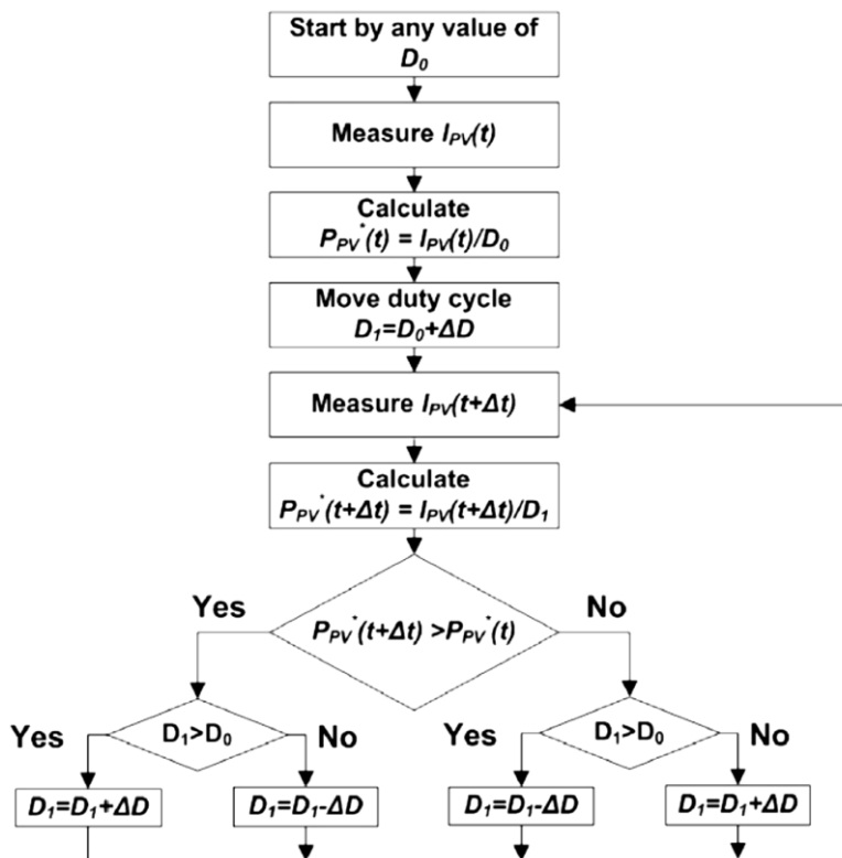
شکل ۱۳: فلچارت روش سلول PV
