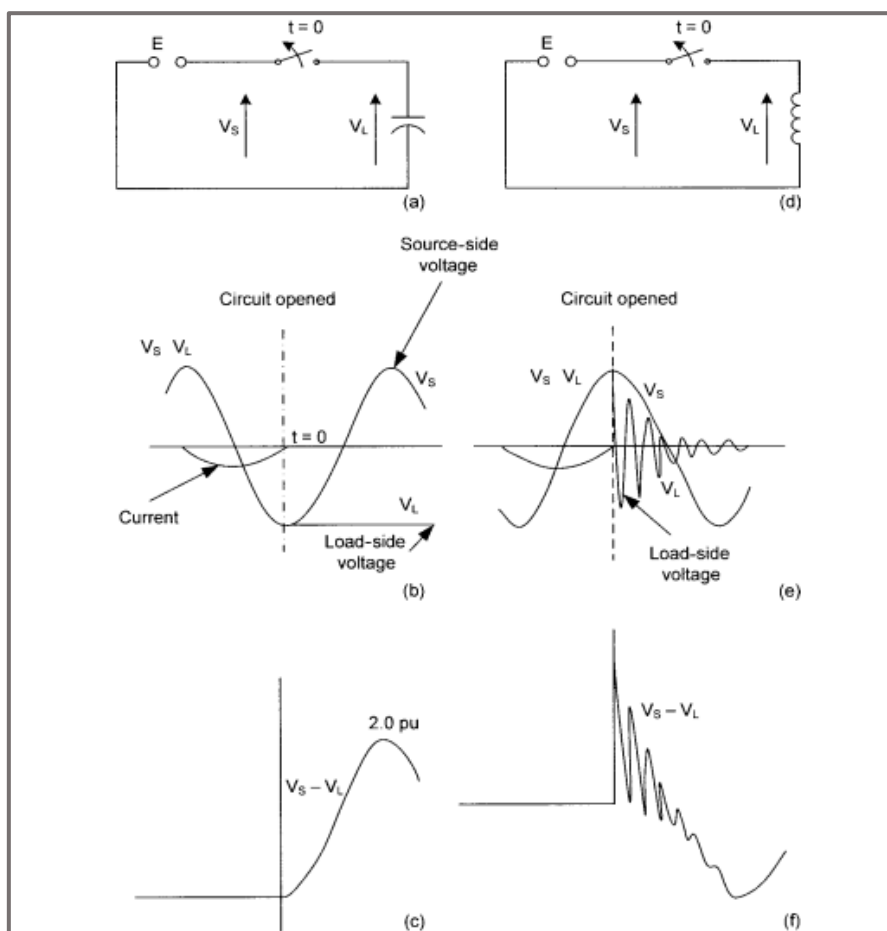
شکل ۱۰: (a)، (b) و (c) به ترتیب قطع جریان خازنی، نمودار مدار ولتاژ سمت بار و منبع و TRV. (d)، (e) و (f) به ترتیب قطع جریان القایی، نمودار مدار ولتاژ سمت بار و منبع و TRV.
