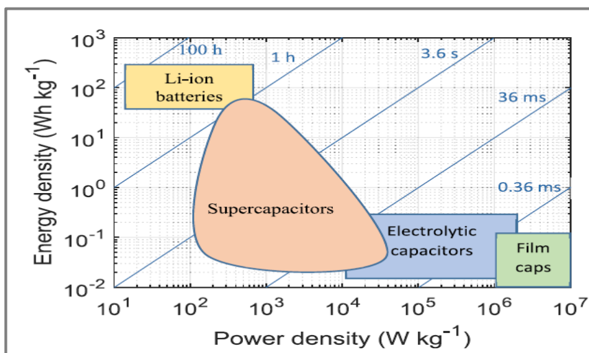
شکل ۱: مشخصه چگالی توان و انرژی انواع ذخیره سازها
