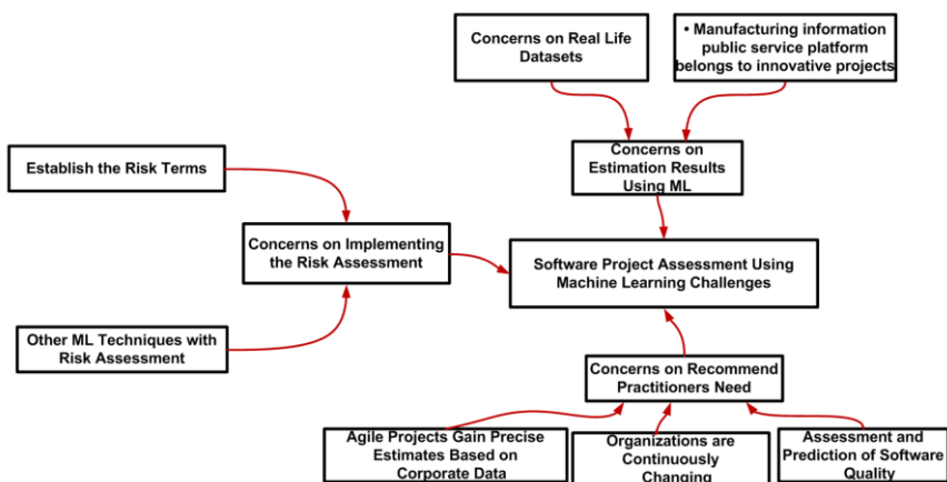
شکل ۷: ارزیابی پروژه نرم‌افزاری با استفاده از چالش‌های یادگیری ماشین
